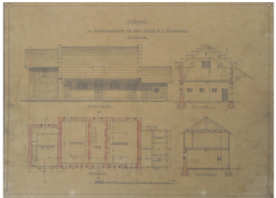
Aufriss, Grund- und Querschnitt für ein Wirtschaftsgebäude von Emil Freiherr von Schauenburg in Gaisbach, um 1850. Vorlage: Archiv der Freiherren von Schauenburg, Oberkirch
